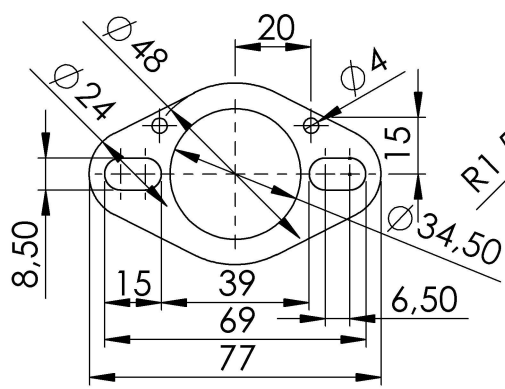
"S.S. flange" Cod.206443
