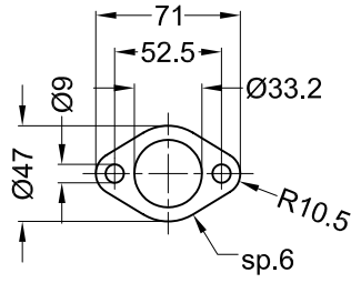
Vista "B" Flangia "43A"
